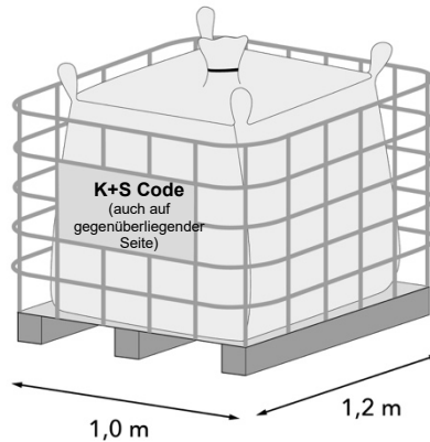
IBC-Gitterbox mit innenliegendem UTD-Big- Bag
