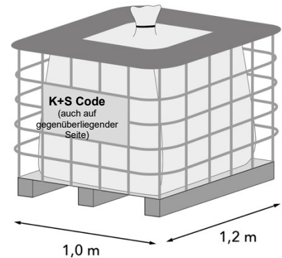
IBC-Gitterbox mit innenliegendem UTD-Big- Bag und aufgesetztem Rahmen
